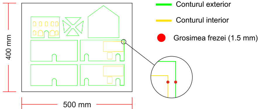
Model de aranjare piese debitare mecanica cnc
